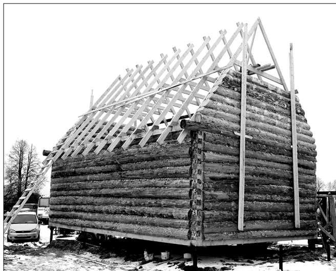
Стропила на срубе часовни
